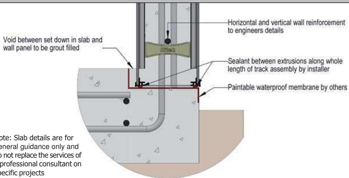
SLAB EDGE DETAIL
