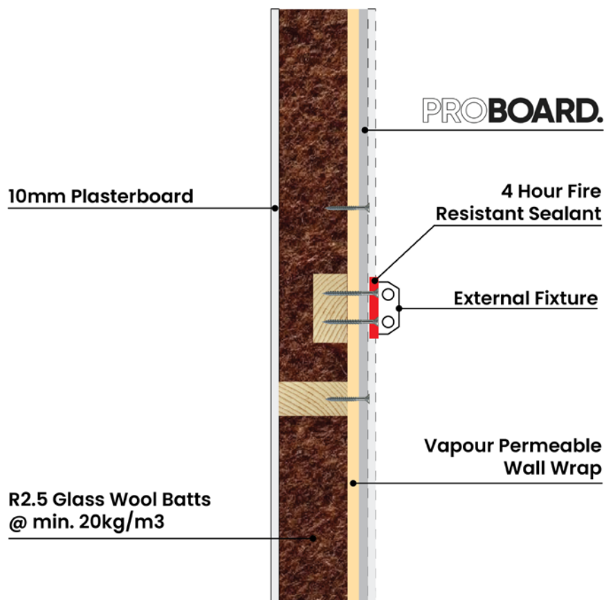
ProBoard External Fixing D19
